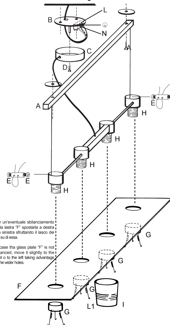
POSIZIONE FINALE DEL BICCHIERINO MOLATO FINAL POSITION OF THE GROUND GLASS
